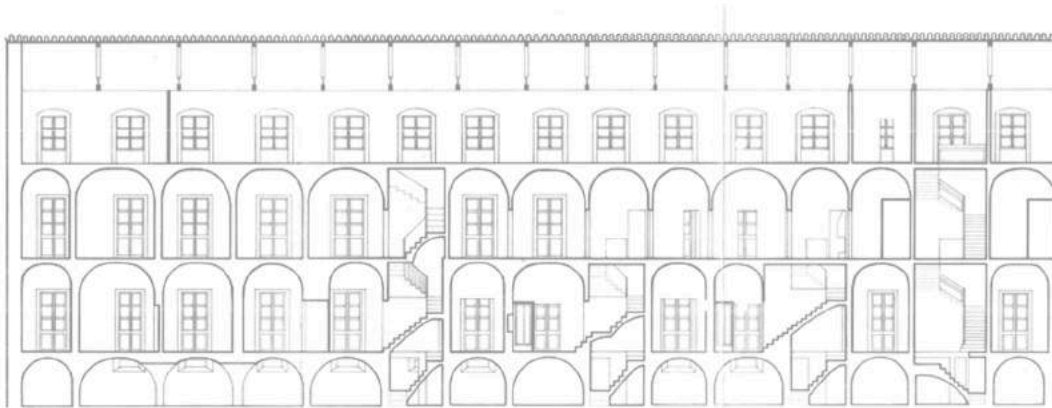
Edifici Claustres. Secció longitudinal.
