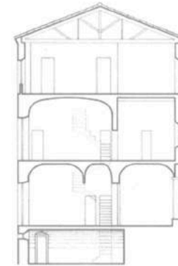
Edifici Claustres. Secció transversal.
