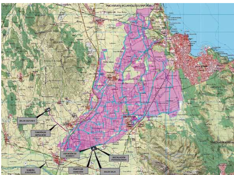
Xarxa de distribució al corredor d'Albons.
