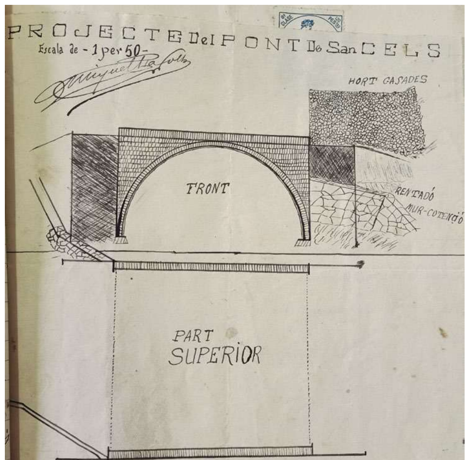
Plànol del projecte del nou pont de Sant Cels.
