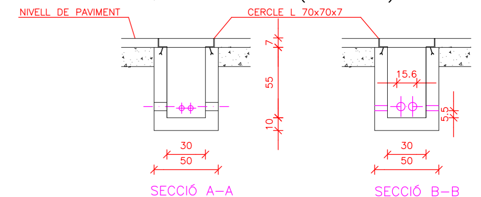
DIMENSIONES DE LA ARQUETA TIPO D PREFABRICADA (HIPOTESIS II-III) CON TAPA DE HORMIGÓN
