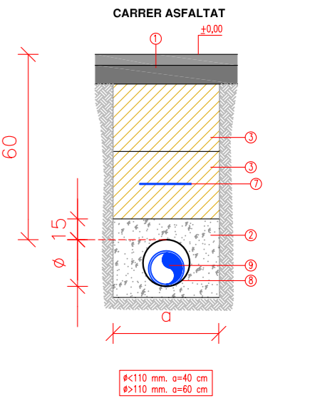
DETALL RASA TIPUS PER A CANALITZAT SOTA VIAL
