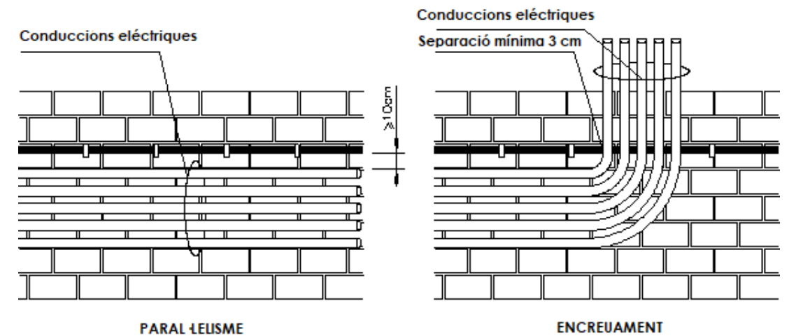
Fig. 18. Distàncies a complir amb conduccions elèctriques
