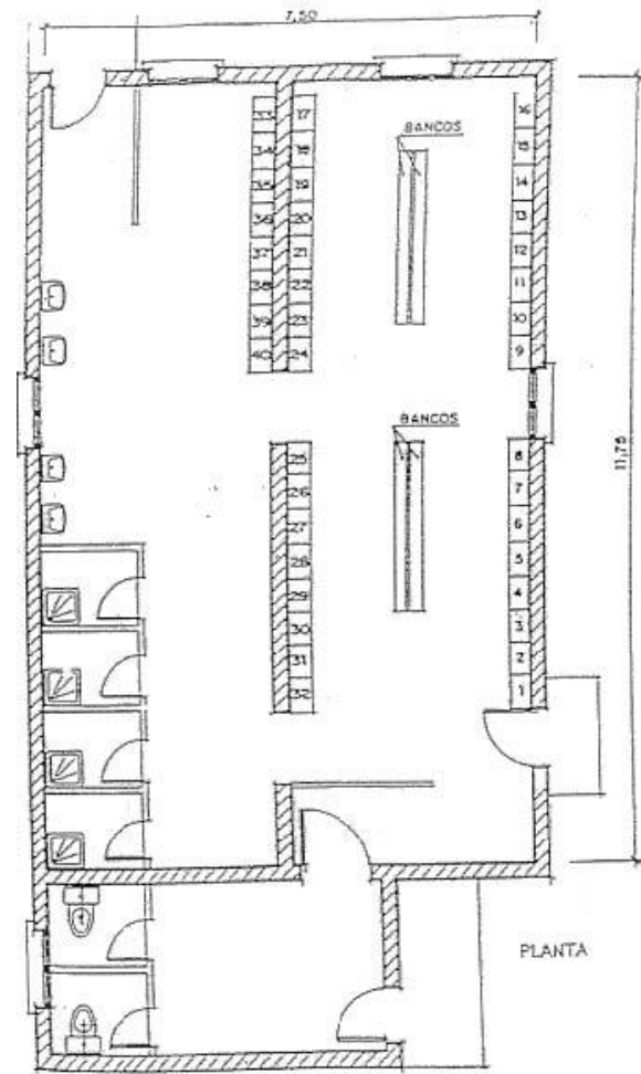
8.17.1.28. CASETA PER A VESTUARIS I SERVEIS
