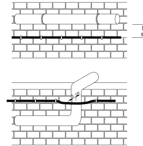
Fig. 17. Distàncies a complir amb canalitzacions de gas
