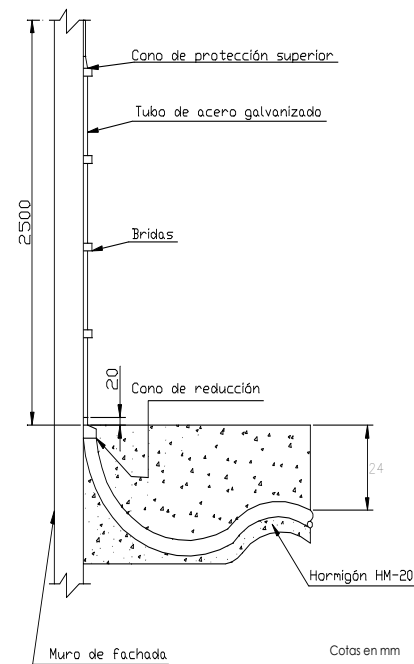
Fig. 3. Secció de sortida a façana
