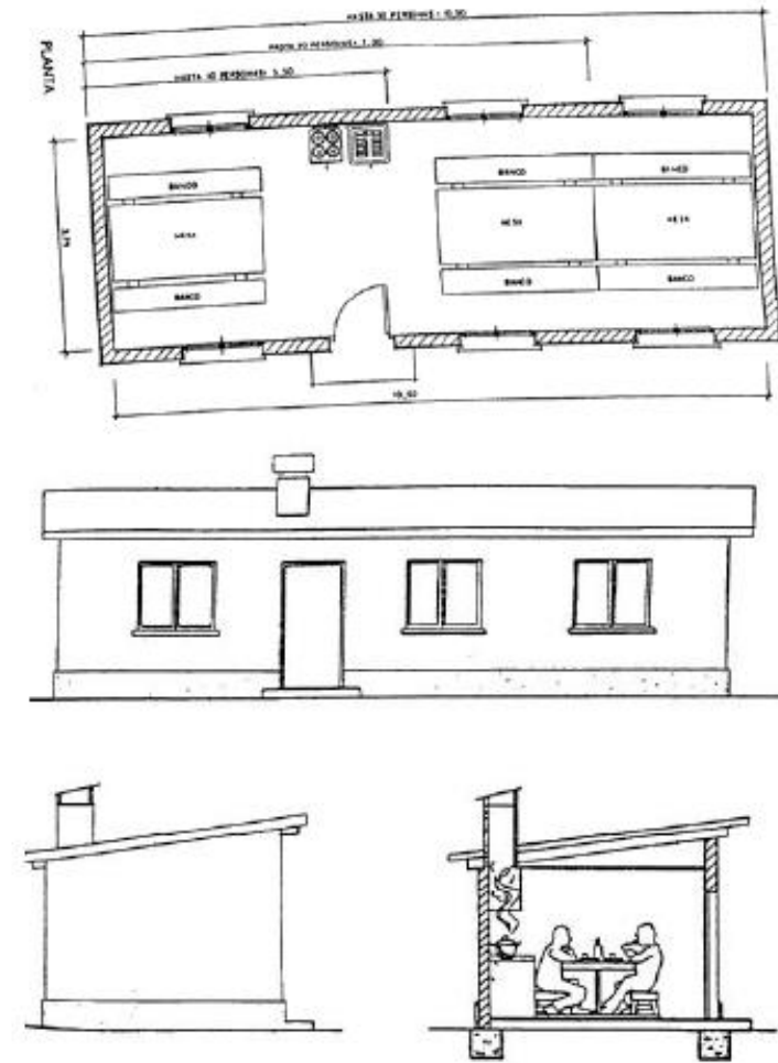
8.17.1.31. CASETA PER A MENJADOR D'OBRA
