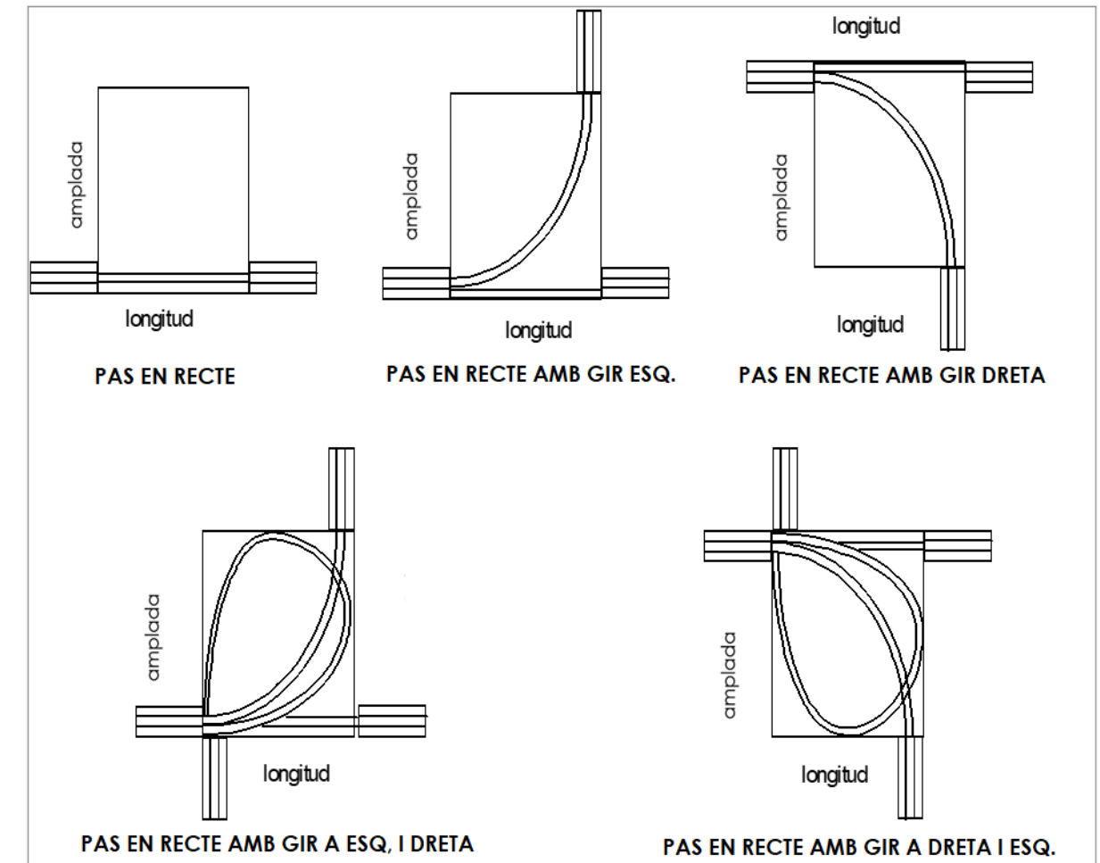
Fig. 2. Possibilitats d'Accés a les Arquetes
