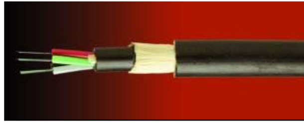
Fig. 4. Exemple de cable de fibra per estesa mixta interior / exterior (tipus TKT)
