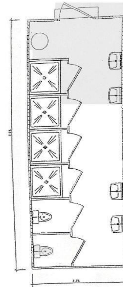
8.17.1.29. CASETA PER A SERVEIS D'OBRA
