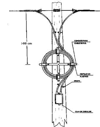
Fig. 22. Instal·lació de caixa d'acoblament a pal
