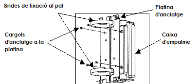
Fig. 21. Detall instal·lació de caixa d'acoblament a pal
