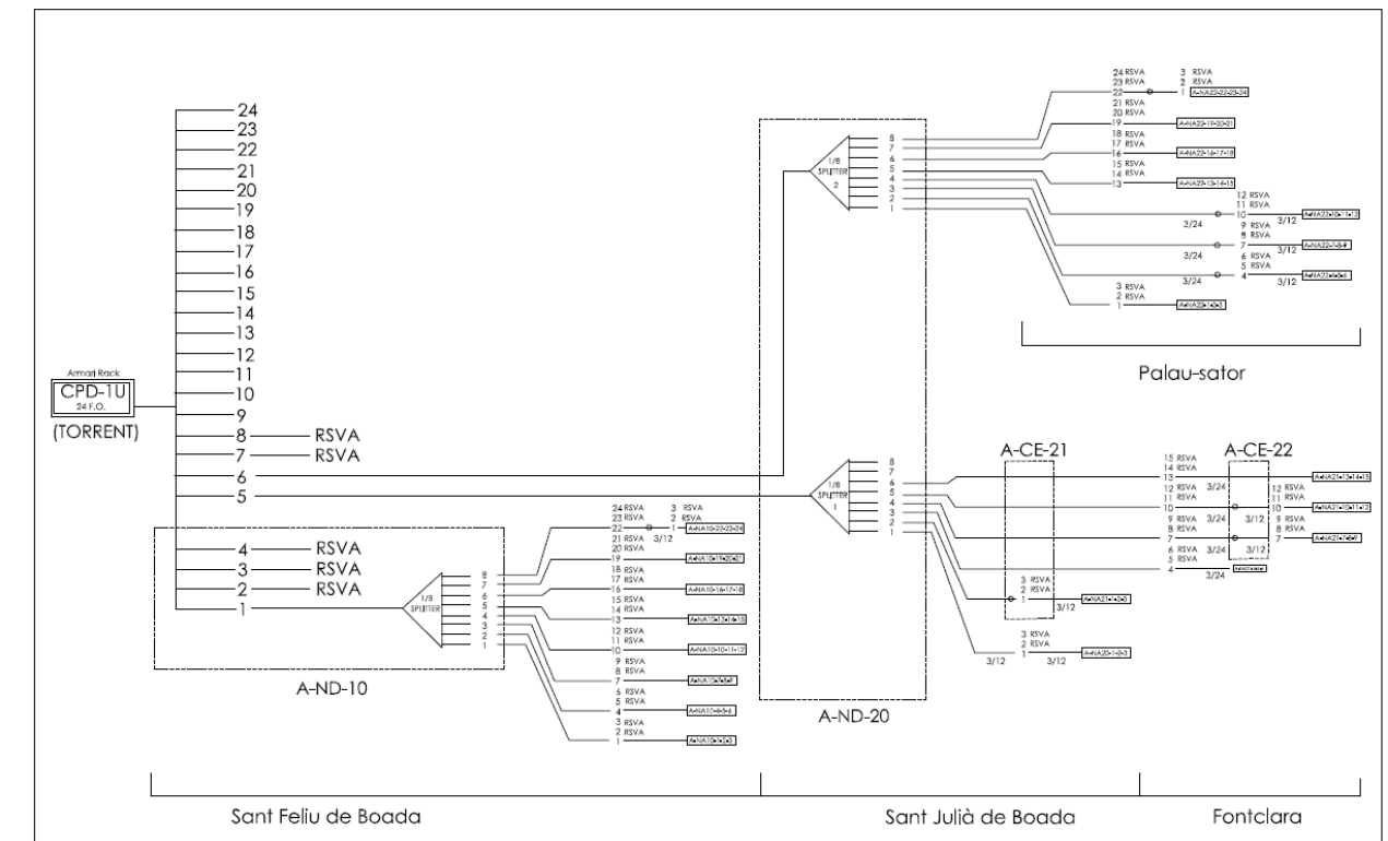
Fig. 1. Distribució interna inicial de la xarxa FTTH.(veure plànols)
