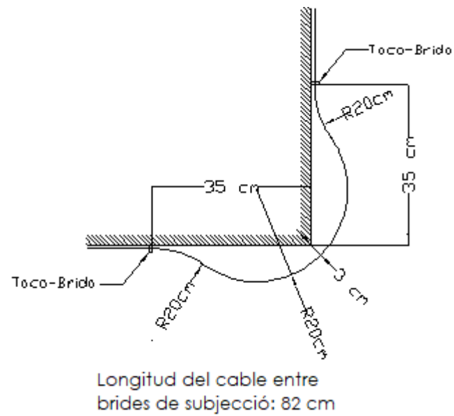
Fig. 16. Esquema de cablejat a cantonades
