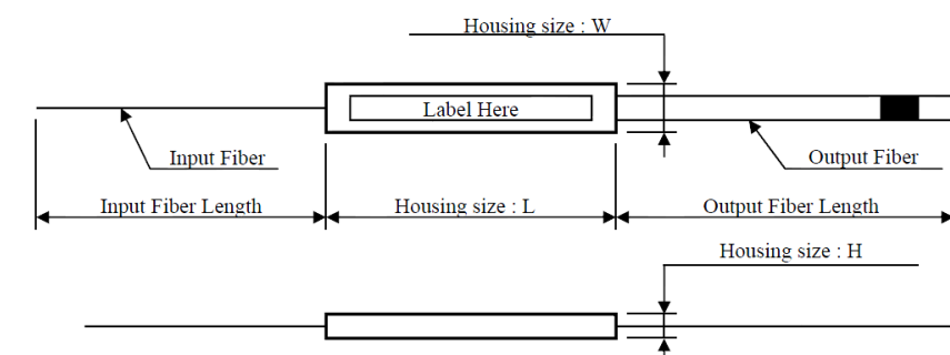
Fig. 9. Exemple de splitter planar 1x8
