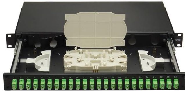
Fig. 10. Exemple de safata al rack
