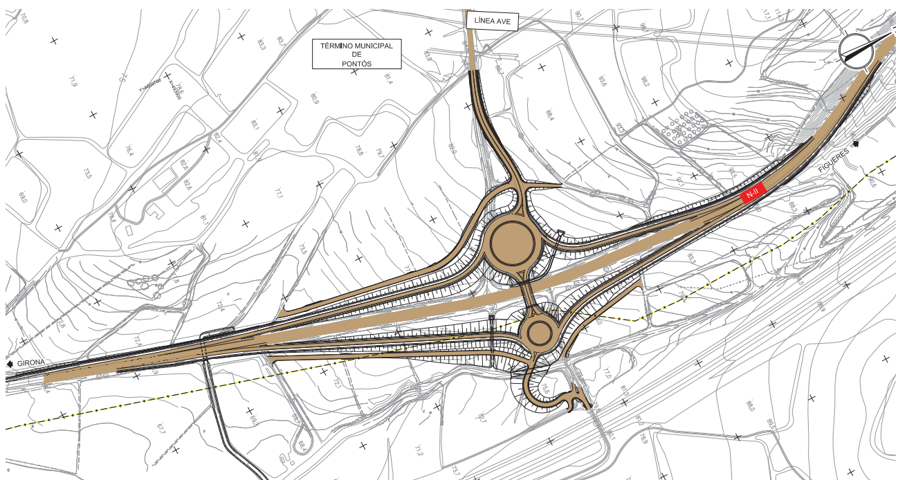
Plànol del projecte de l'enllaç de Pontós des de la carretera N-II
