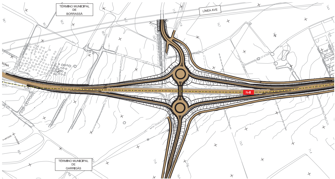
Plànol del projecte de l'enllaç de Garrigàs i Creixell des de la carretera N-II
