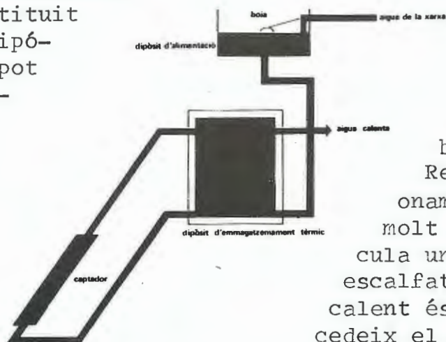
Figura 12. Esquema bàsic d'una instal·lació solar productora d'aigua calenta sanitària.
