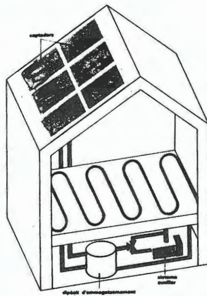
Figura 16. Instal·lació d'energia solar per a calefacció mitjançant terra radiant.
