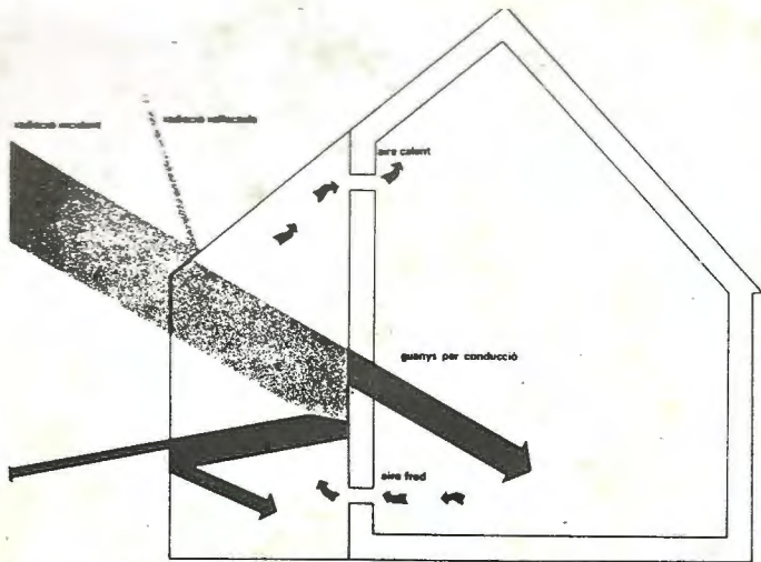
Figura 7. Distribució dels fluxos d'energia en un hivernacle.
