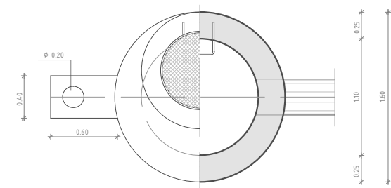
SECCIÓ E 1 : 50
