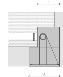
SECCIÓ A-A
