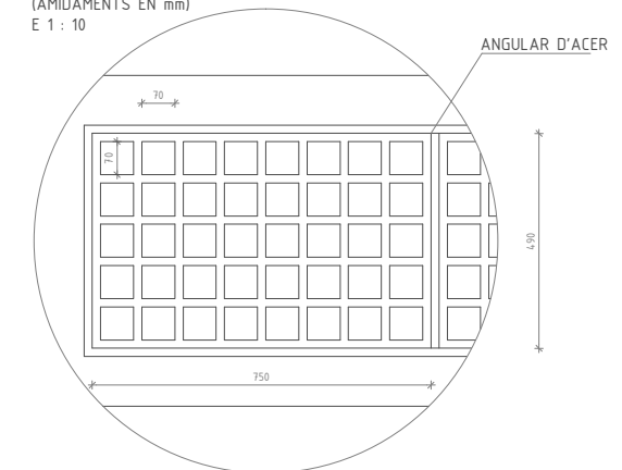
POU DE RESALT PLANTA E 1 : 50
