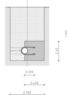
SECCIÓ
