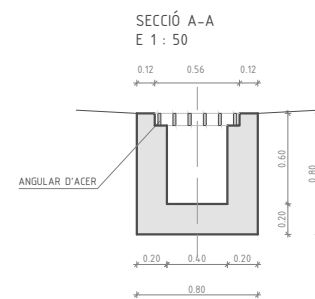
SECCIÓ TIPUS CONDUCTE E 1 : 50
