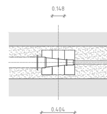
CON DE REDUCCIÓ PLANTA
