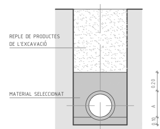
SECCIÓ TIPUS CONDUCTE AMB CANONADA PROTEGIDA E 1 : 50
