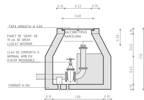
SECCIÓ E 1 : 40
