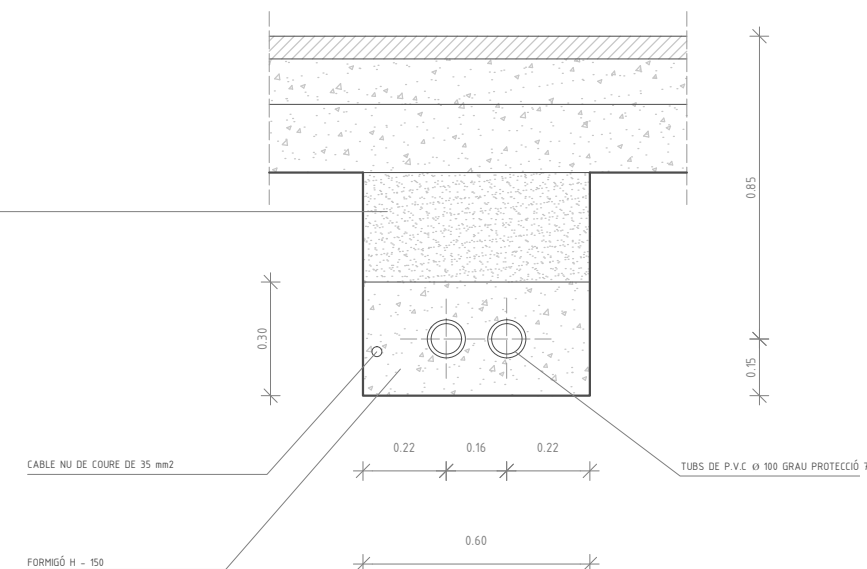
CABLES A ZONA DE VIALS E: 1 : 20
