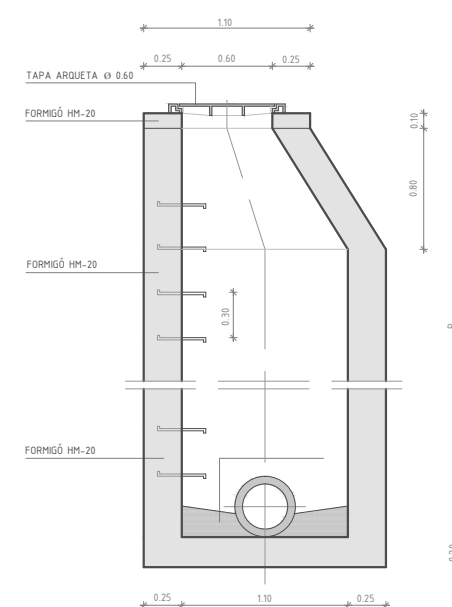
SECCIÓ E 1 : 50
