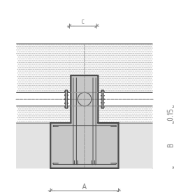
SECCIÓ B-B
