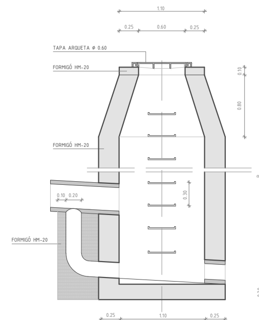
SECCIÓ E 1 : 50
