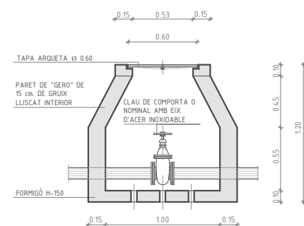
SECCIÓ E 1 : 40
