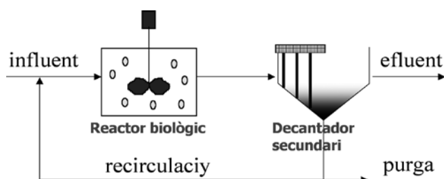
Figura 3. Esquema general dels fluxos en una depuradora
